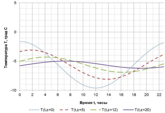
Рисунок 3 – Зміна температури в шарах дорожнього одягу в зимовий період Figure 3 – Change in temperature in the layers of road pavement in the winter
